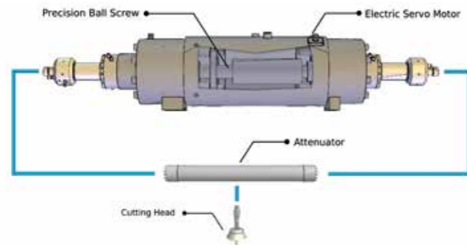
Multiplicador de pressão de ação dupla, de acionamento elétrico, feito de alta resistência mecânica e material anticorrosivo.
